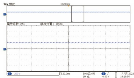
IEC61000-4-17直流纹波
