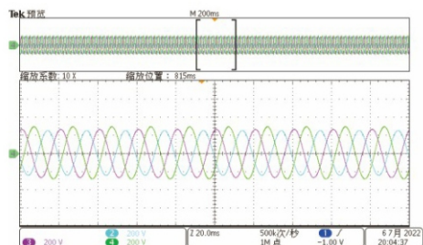
IEC61000-4-27电压不平衡
