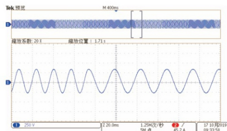
IEC61000-4-28工频频率变化
