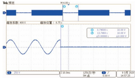
IEC61000-4-11电压暂降
